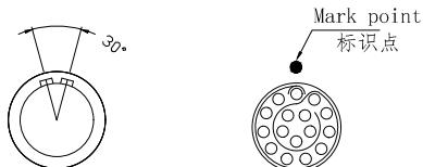
插头前视图
