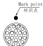
K向孔位排列
