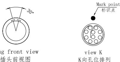
K向孔位排列
